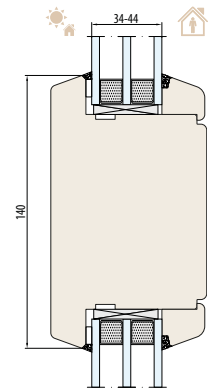
SYSTEM NATURO 80 Konstruktionsprosse 140 mm
