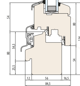
SYSTEM NATURO 68 Äußere Fensterbankfräsung
