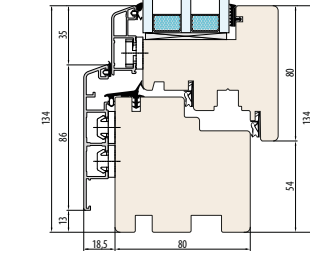
SYSTEM NATURO 80 ALU GEMINI CLASSIC Ohne Fensterbankfräsung
