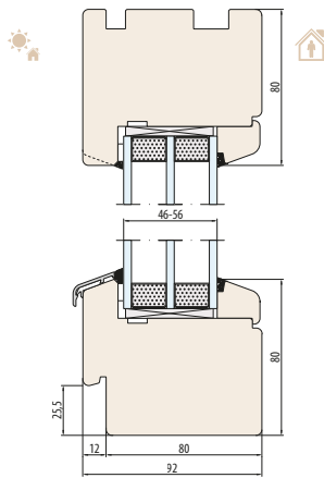
SYSTEM NATURO 92-Fix Äußere Fensterbankfräsung
