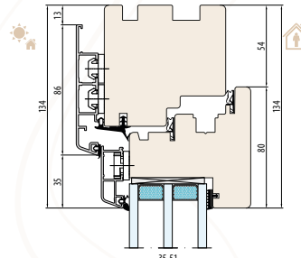
SYSTEM NATURO 80 ALU GEMINI CLASSIC Innen- und Außenfensterbankfräsung
