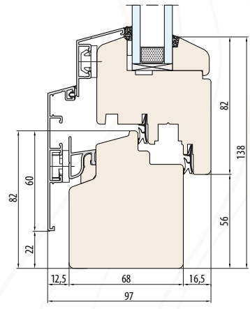
SYSTEM NATURO 68 ALU RENO LINE ohne Fensterbankfräsung
