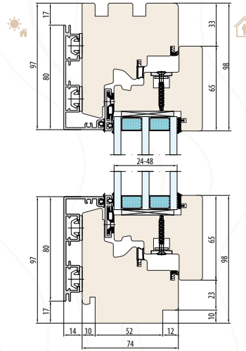
SYSTEM ESPERIA LIFE 74 ALU Innen- und Außenfensterbankfräsung
