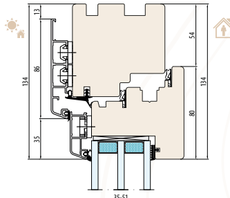
SYSTEM NATURO 80 ALU GEMINI CLASSIC Ohne Fensterbankfräsung
