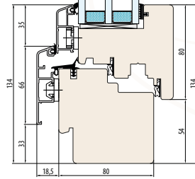
SYSTEM NATURO 80 ALU GEMINI CLASSIC Äußere Fensterbankfräsung
