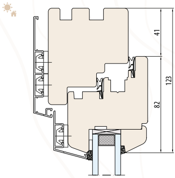
VERTIKALSCHNITT A-A
