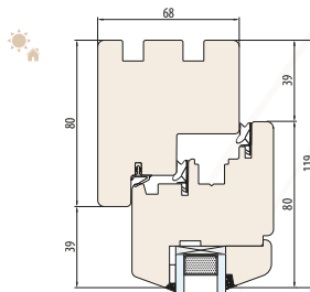
SYSTEM NATURO 68 Ohne Fensterbankfräsung
