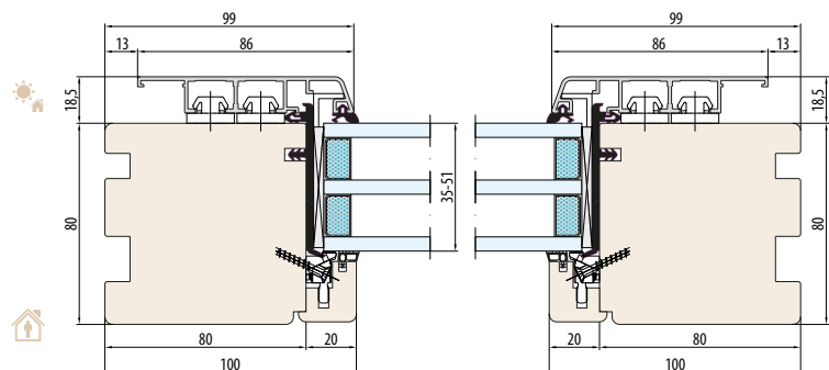
HORIZONTALSCHNITT B-B
