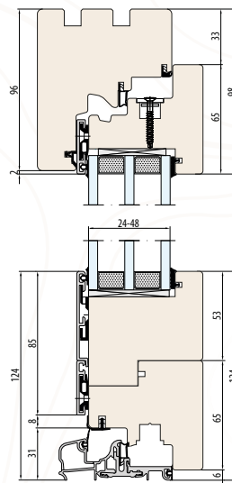
SYSTEM ESPERIA LIFE 80 Einfügelige Balkontüren mit niedriger Schwelle
