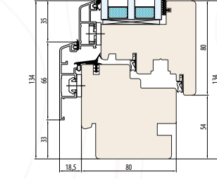
SYSTEM NATURO 80 ALU GEMINI CLASSIC Innen- und Außenfensterbankfräsung
