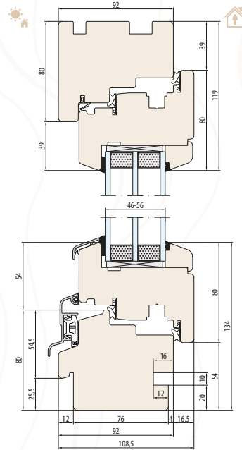
SYSTEM NATURO 92 Innen- und Außenfensterbankfräsung
