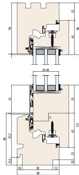
SYSTEM ESPERIA LIFE 80 Einfügelige Balkontüren mit hoher Schwelle
