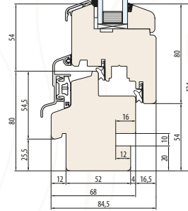
SYSTEM NATURO 68 Innen- und Außenfensterbankfräsung
