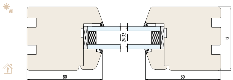
SYSTEM NATURO 68-Fix HORIZONTALSCHNITT B-B
