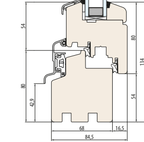
SYSTEM NATURO 68 Ohne Fensterbankfräsung
