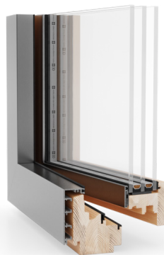
Standardprofil (mit Fensterbankkräsung)
