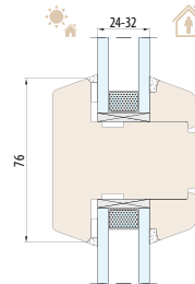
SYSTEM NATURO 68 Konstruktionsprosse 76 mm
