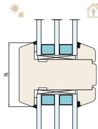
SYSTEM NATURO 92 Konstruktionssprosse 76 mm
