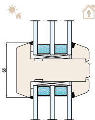
SYSTEM NATURO 92 Konstruktionssprosse 68 mm
